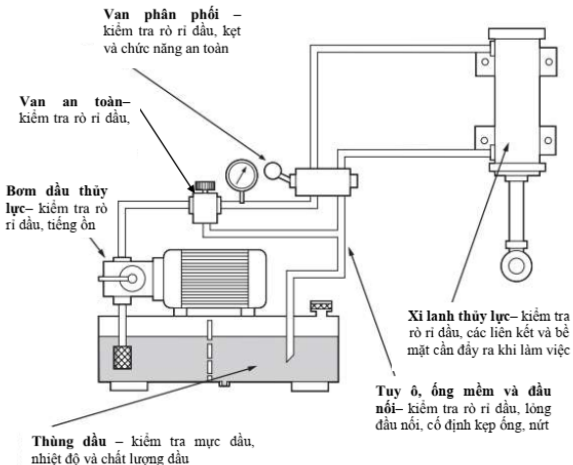
Hình B.1 Sơ đồ hệ thống dẫn động thủy lực máy ép cọc với các phần tử thủy lực được coi là quan trọng (theo quan điểm kỹ thuật an toàn) và chỉ dẫn kiểm tra rò rỉ bên ngoài bằng trực quan
