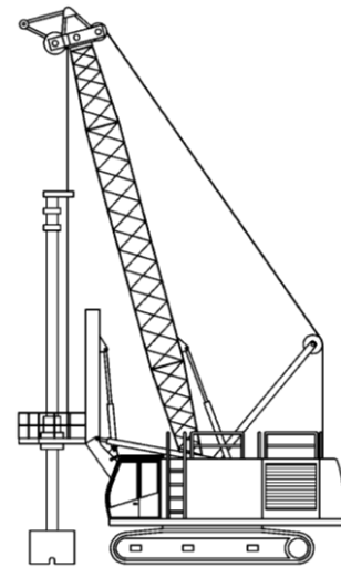
Hình A.1.2.3 Máy khoan cọc nhồi với máy khoan gắn trên cần trục tự hành.
