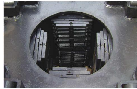
Hình A.2.2.3 Hộp kẹp cọc với chấu kẹp cọc phẳng dùng để ép cọc vuông
