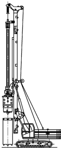
Hình A.1.2.2 Máy khoan cọc nhồi với máy khoan cần Kelly.
