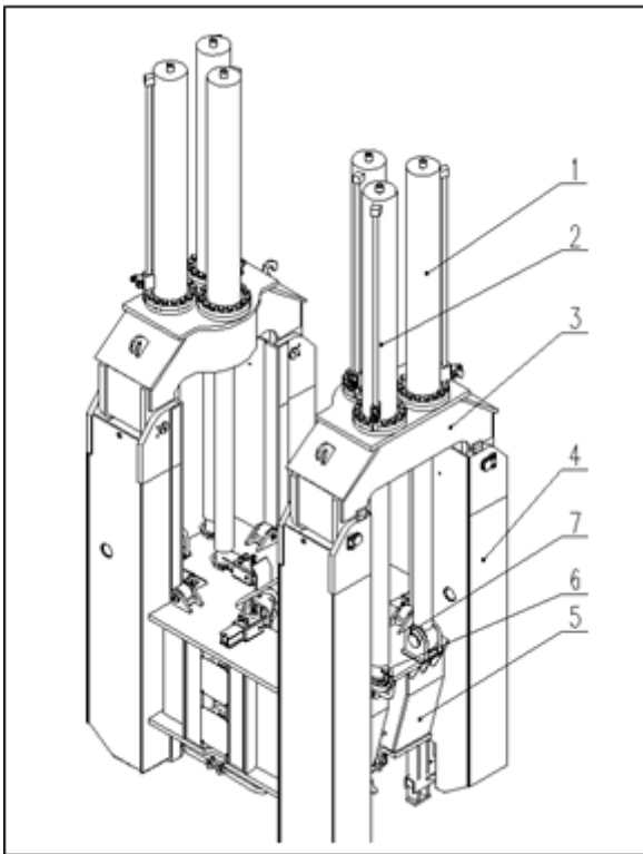
Hình A.2.2.2 Cấu tạo của cơ cấu ép cọc: 1, 2 – Các xi lanh thủy lực ép cọc (chính và phụ); 3 – dầm ngang đỡ các xi lanh thủy lực ép cọc; 4 – trụ đứng dẫn hướng ép cọc; 5- hộp kẹp cọc; 6 - ắc và chốt ghép cần của xi lanh thủy lực ép cọc với hộp kẹp cọc; 7 – Bát cầu trên hộp kẹp cọc có nhiệm vụ tiếp nhận đầu dạng cầu tròn của các xi lanh thủy lực ép cọc phụ
