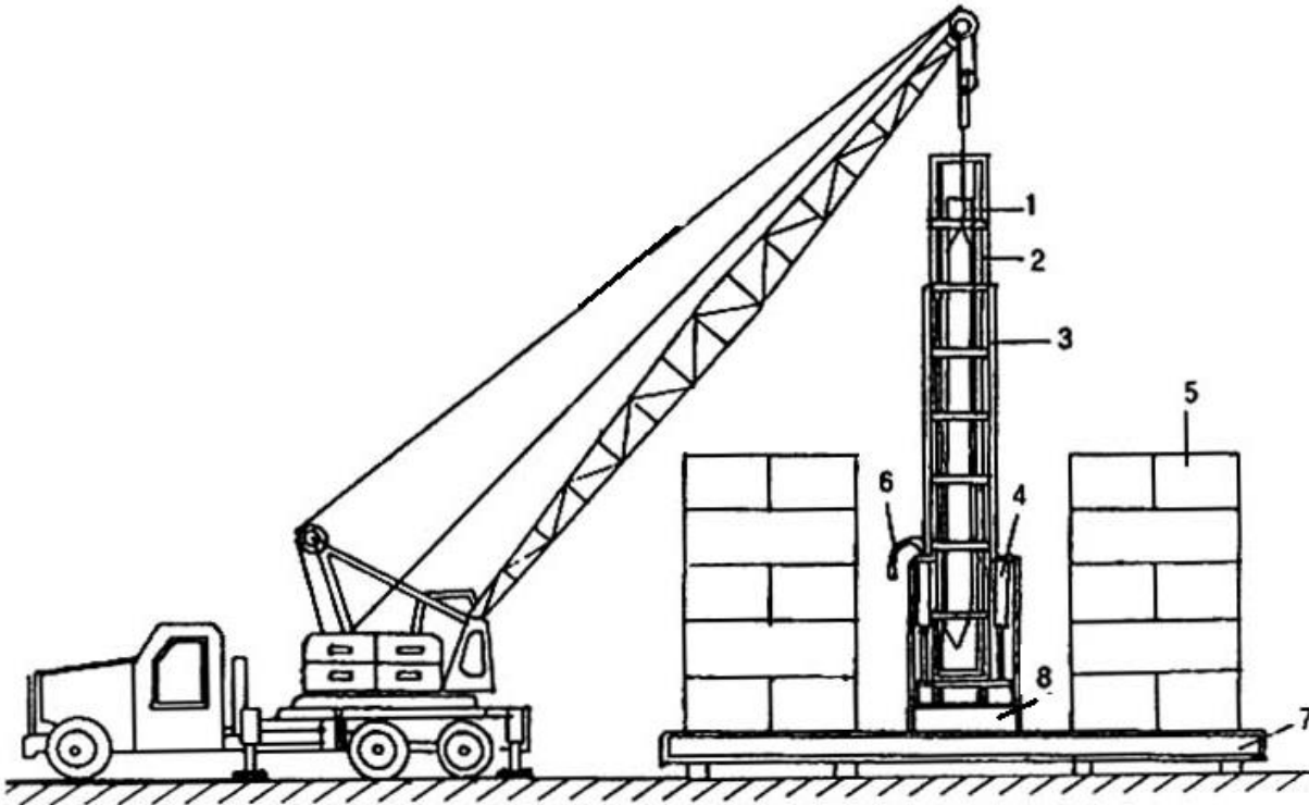
Hình A.2.1 Máy ép tải loại ép đỉnh (ép chặn): 1 – cọc ép; 2 – khung dẫn hướng di động; 3 – khung dẫn hướng cố định; 4 - Xi lanh ép; 5 - đối trọng (tải); 6 – ống mềm dẫn dầu thủy lực; 7 – khung chính; 8 – khung phụ
