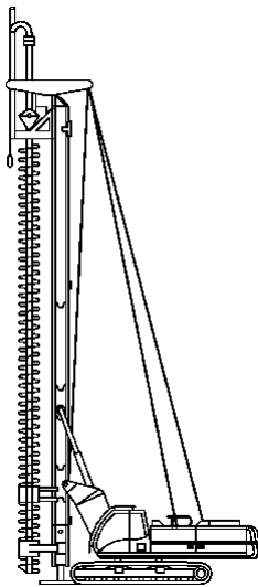
Hình A.1.2.1 Máy khoan cọc nhồi với mũi khoan dạng vít liên tục (CFA) hoặc đầu khoan và vít khoan.
