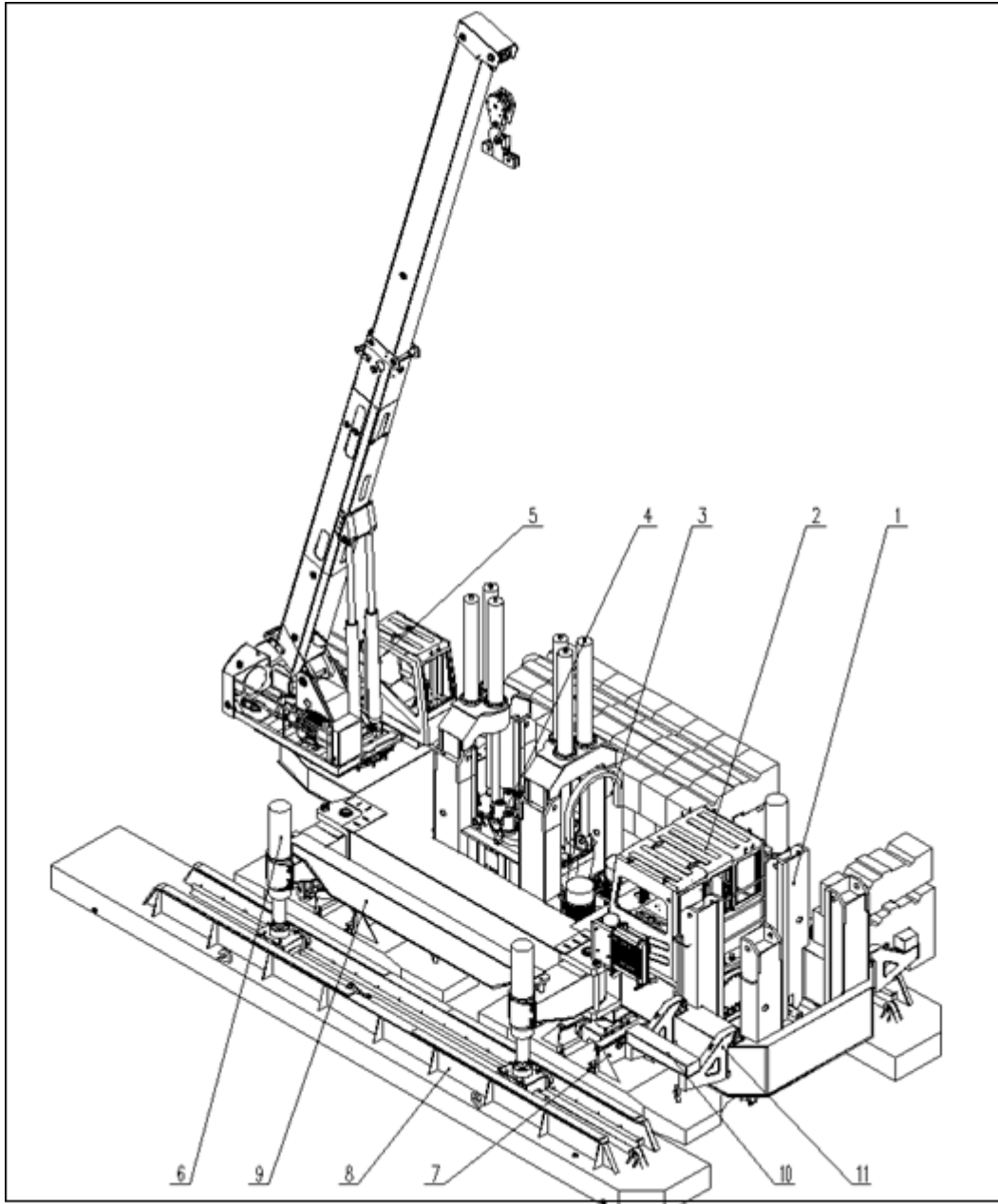
Hình A.2.2.1 Cấu tạo của máy ép ôm loại tự bước: 1 - Cơ cấu ép cạnh: dùng để ép cọc gần các công trình hiện hữu; 2 - Ca bin điều khiển ép cọc; 3 - Cơ cấu ép trung tâm (cơ cấu ép chính); 4 – hộp kẹp cọc: có nhiệm vụ kẹp cọc; 5 - Cần trục: dùng để cẩu các kết cấu máy, cọc, các cục đối trọng; 6 - Các xi lanh thủy lực đỡ bàn máy (cơ cấu nâng hạ máy theo phương thẳng đứng); 7 - Cơ cấu di chuyển ngang và quay: có nhiệm vụ di chuyển máy theo phương vuông góc với phương dọc của máy hoặc quay máy khi di chuyển trên công trường; 8 - Cơ cấu di chuyển dọc: có nhiệm vụ di chuyển máy theo phương dọc của máy khi di chuyển trên công trường; 9 - dầm đỡ đối trọng; 10, 11 - Bàn máy.
