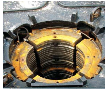
Hình A.2.2.4 Hộp kẹp cọc với chấu kẹp cọc tròn dùng để ép cọc tròn
